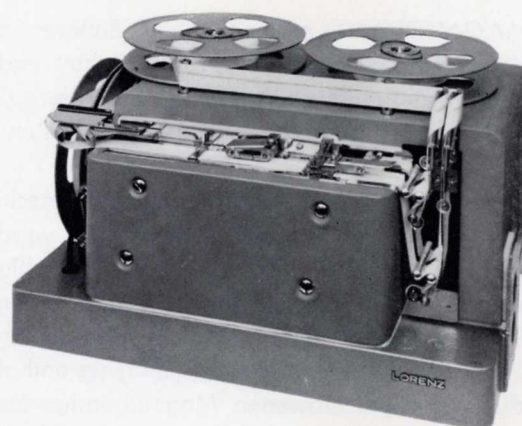
Lochstreifenstanzer SL 614
