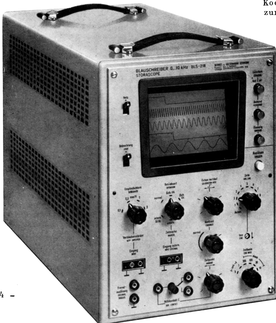
Blauschreiber zur ZUSE Z 23
